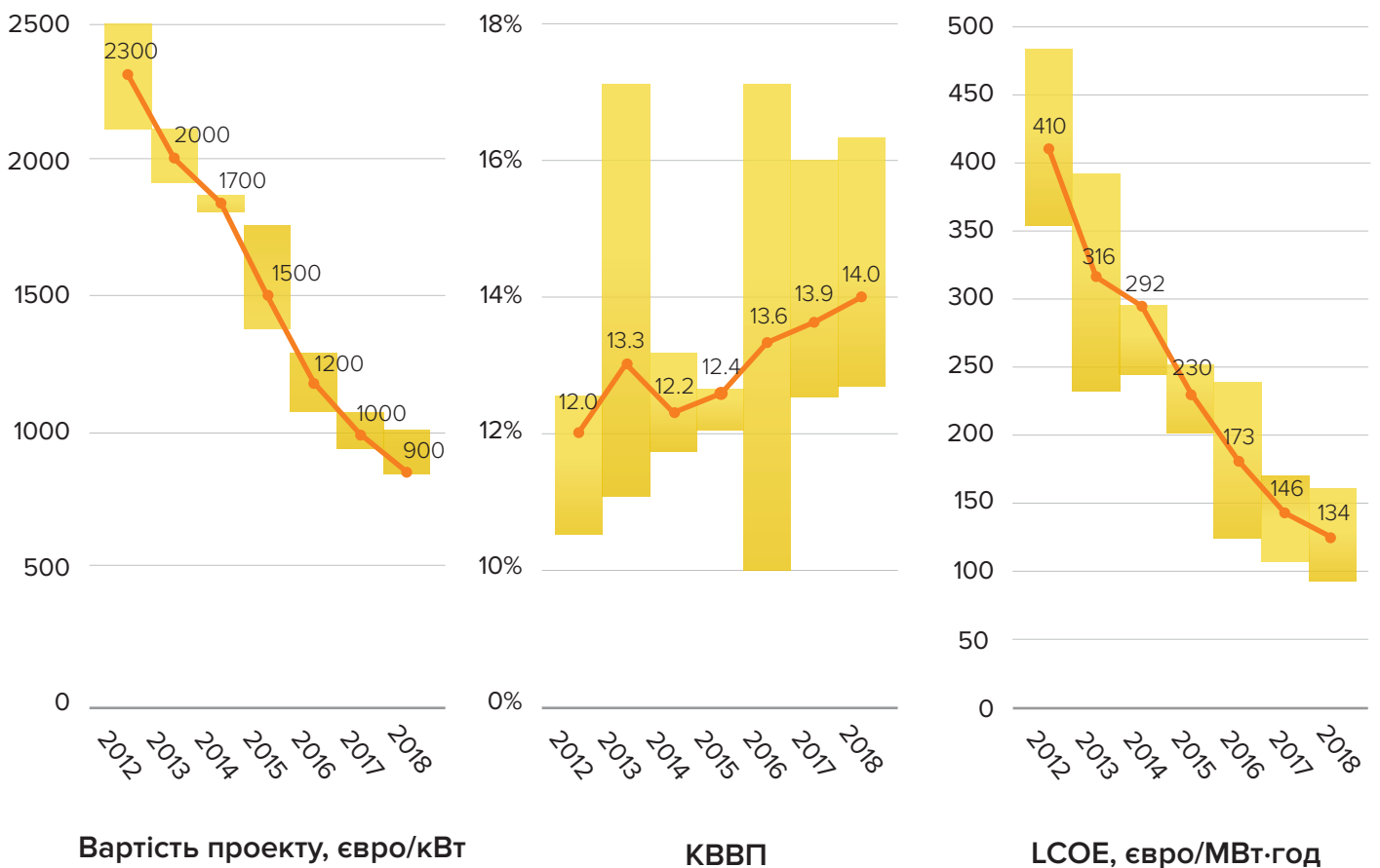
Діаграма 5. LCOE дахових СЕС
