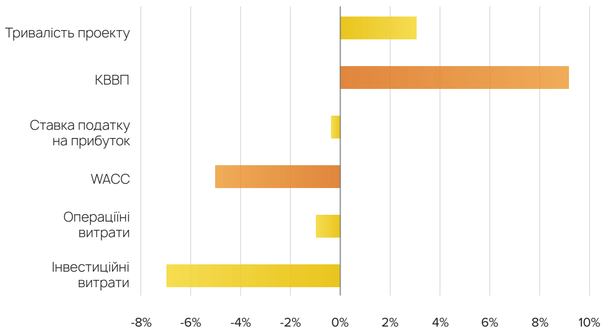
Діаграма 1. Вплив параметрів на LCOE на прикладі СЕС
