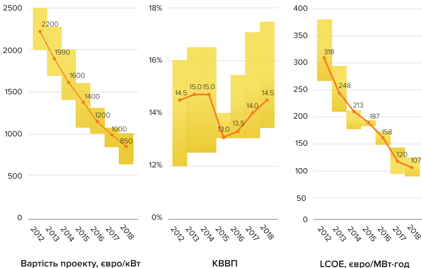
Діаграма 3. LCOE наземних СЕС
