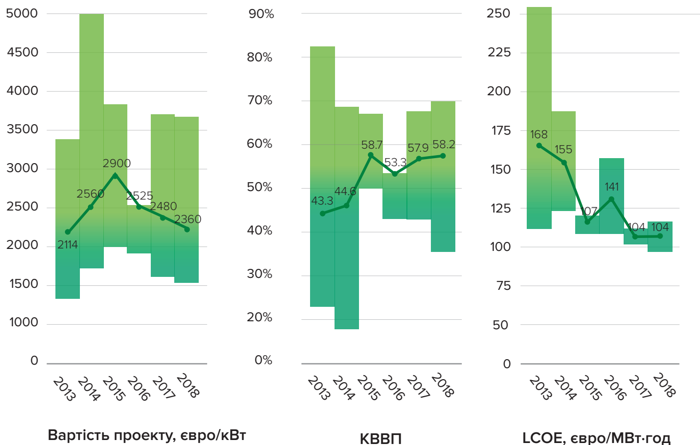
Діаграма 9. LCOE біоенергетичних установок
