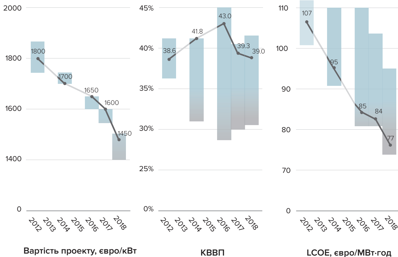
Діаграма 7. LCOE наземних ВЕС
