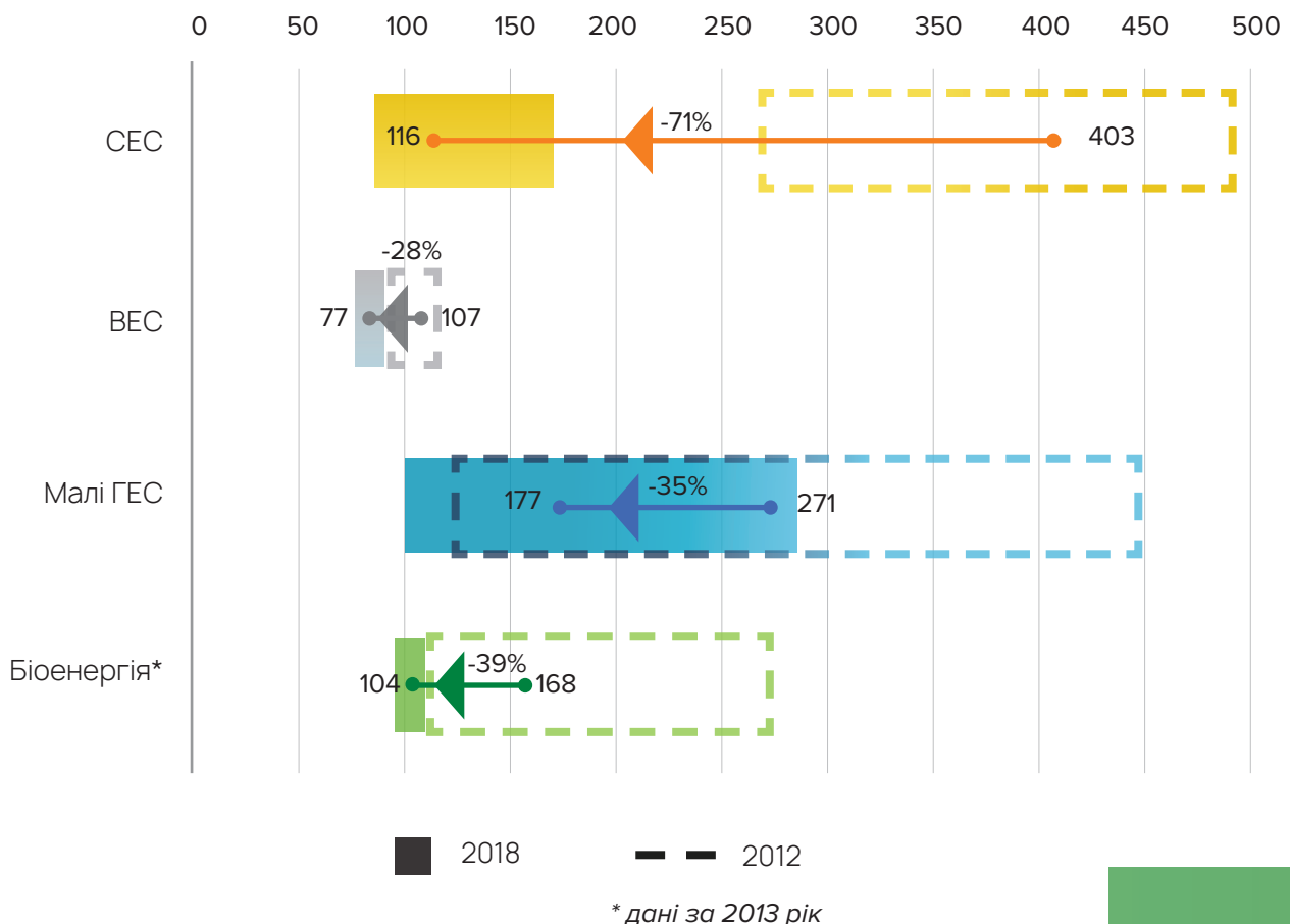
Діаграма А. LCOE основних ВДЕ в Україні, евро/МВт·год
