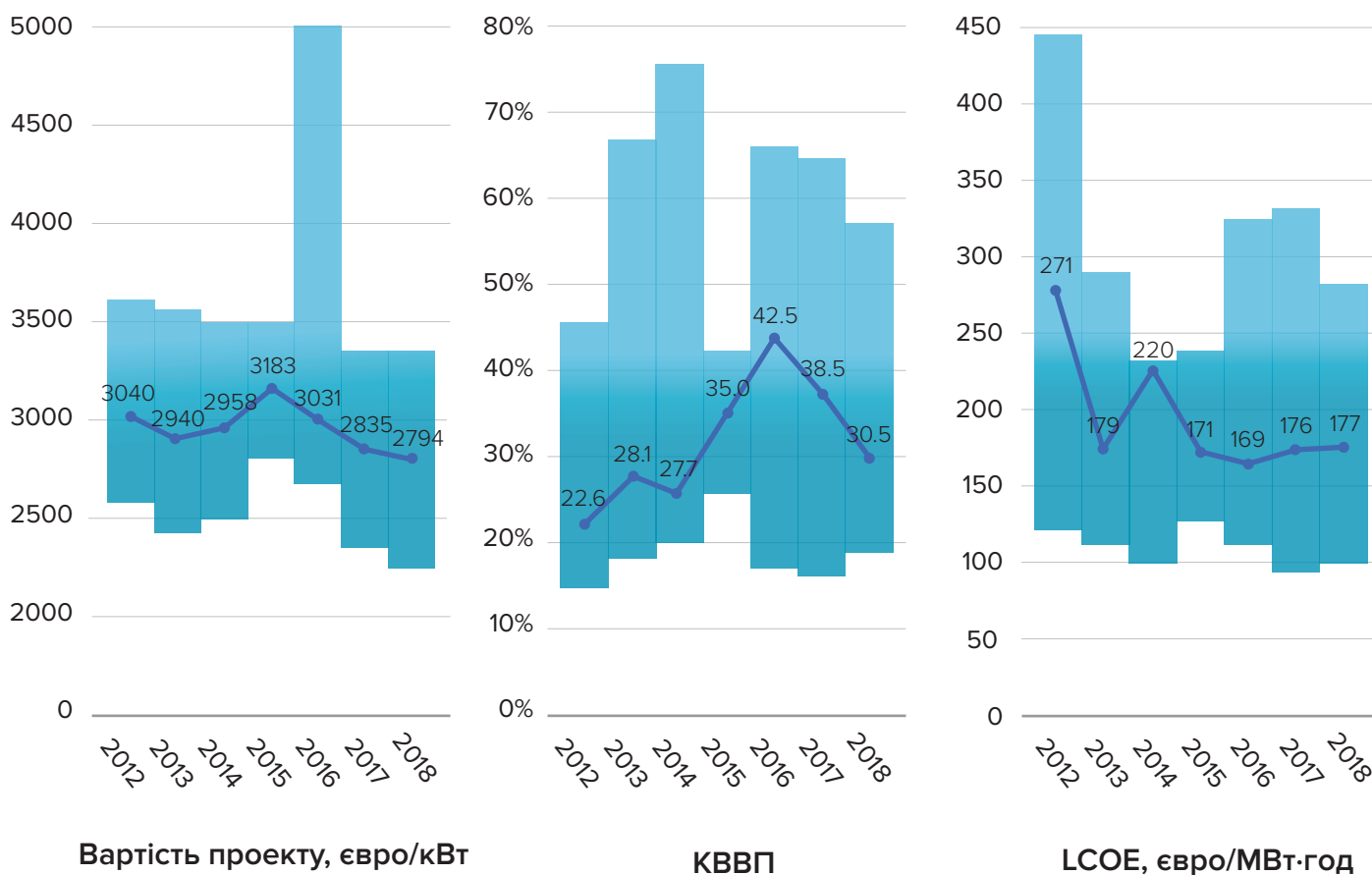
Діаграма 8. LCOE малих ГЕС
